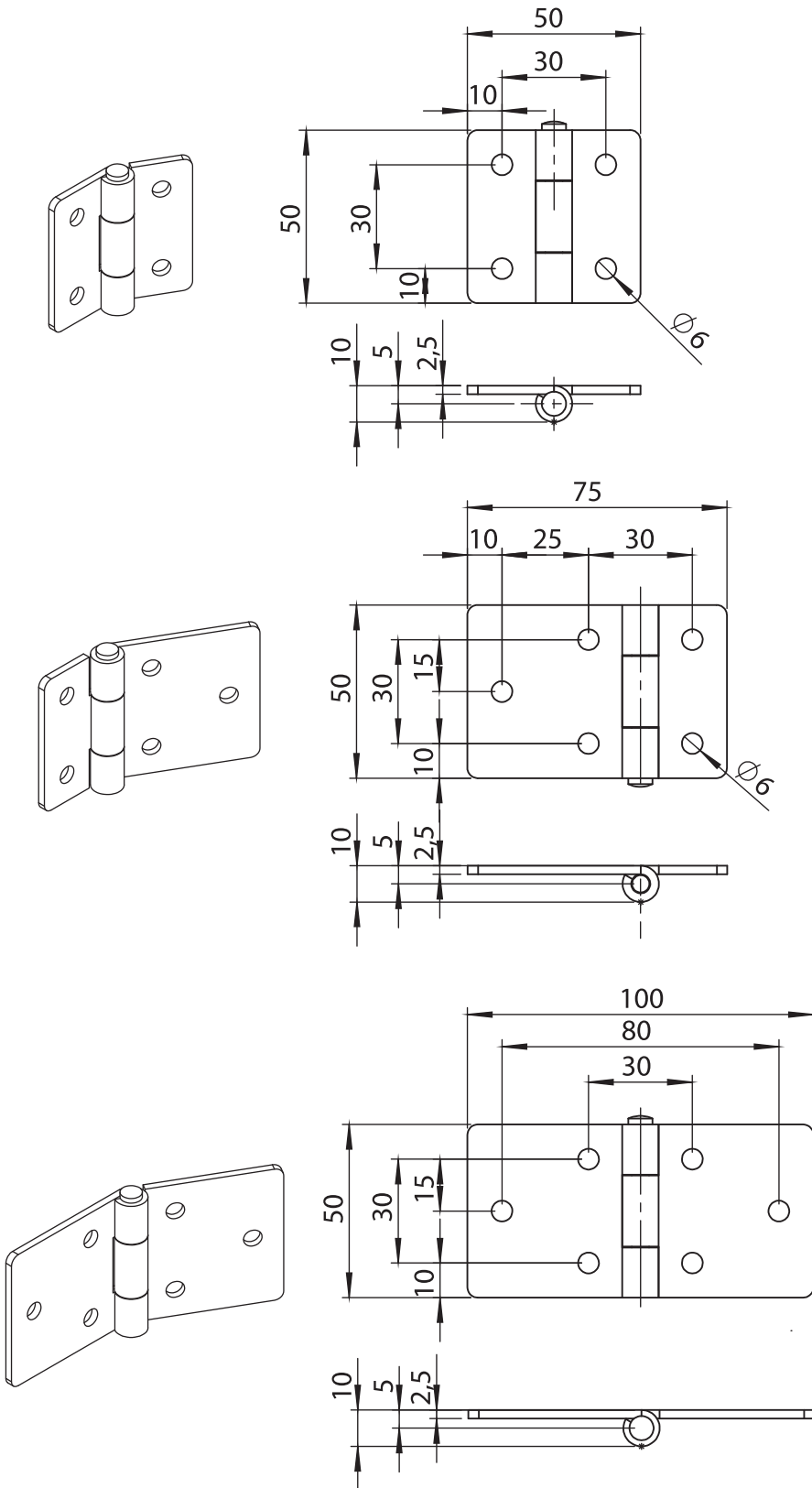
3012 - 180° Hinge
