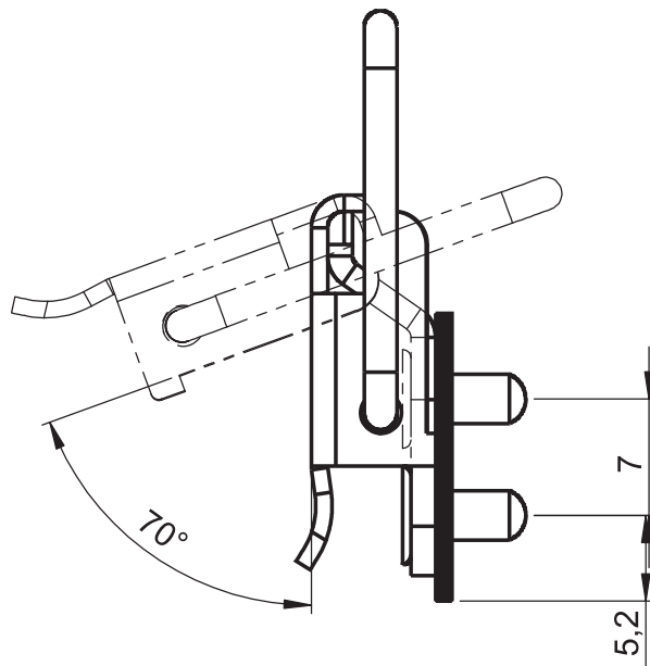
7407 - Toggle Latch
